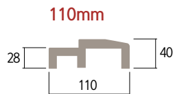
문틀 규격 [단위:mm]
