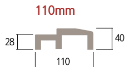
문틀 규격 [단위:mm]
